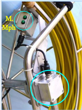
Odomètre ; R à Z ; Affichage en Feet ou Mètres
